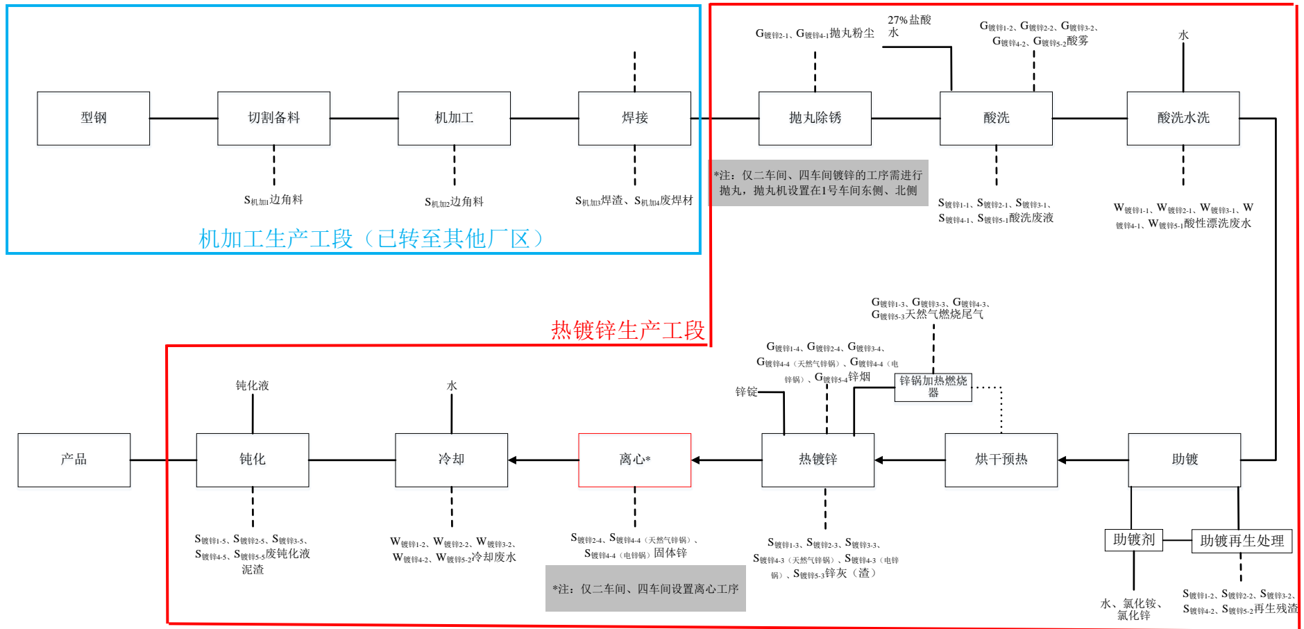
图 3.2-1 金属结构件生产工艺流程及产污环节图
